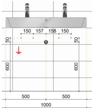
Afvoer/toevoer wastafel
